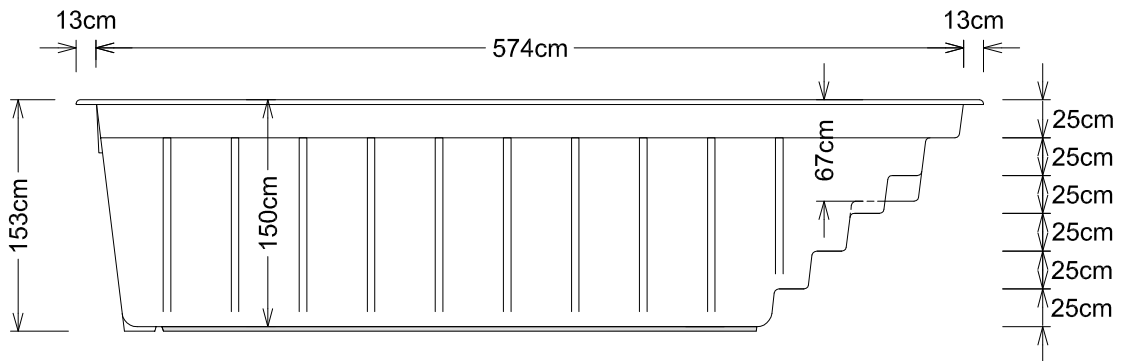
Seitenansicht - Prospetto laterale
