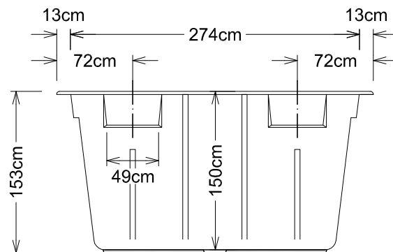
Ansicht Skimmerseite - Prospetto parte Skimmer
