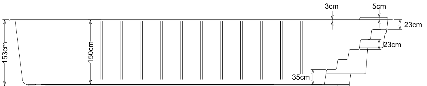
Seitenansicht - Prospetto laterale
