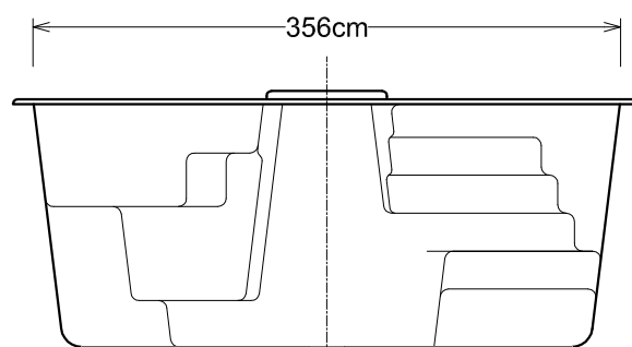
Innenansicht Treppenseite - Prospetto interno parte scala
