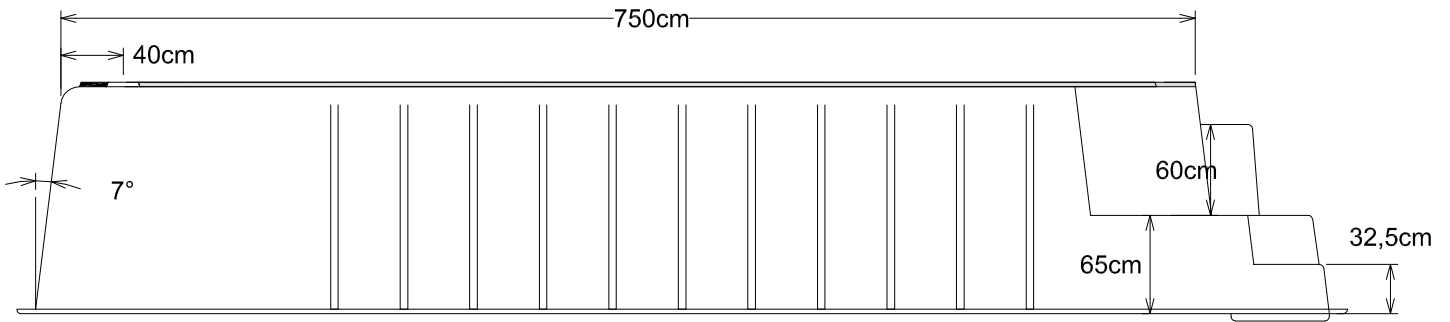
Seitenansicht - Prospetto laterale
